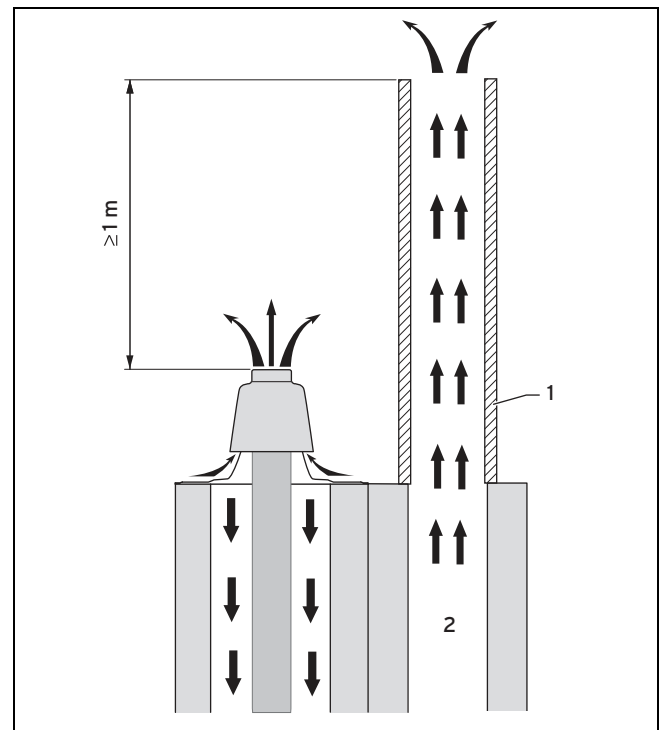
1 Насадка димаря 2 Топочні гази
