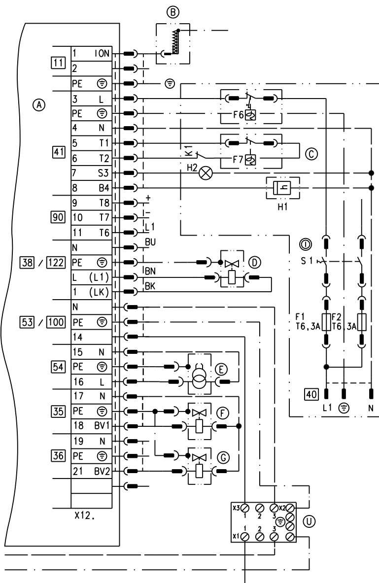
А Топочный автомат VUC 310
