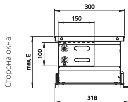
Разрез, высота канала 150/200 мм (пример с рулонной решеткой)
