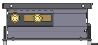
Katherm NK 300
