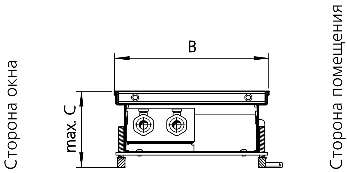
Вид в разрезе, подключение слева, пример NK 232
