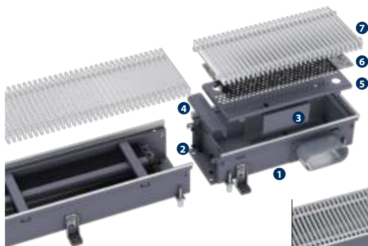
Комбинация Katherm QK с модулем приточного воздуха
