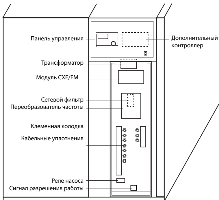
Рис. 16 Передняя панель
