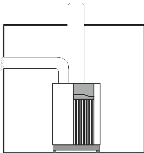
Рис. 18 Горизонтальный воздуховод
