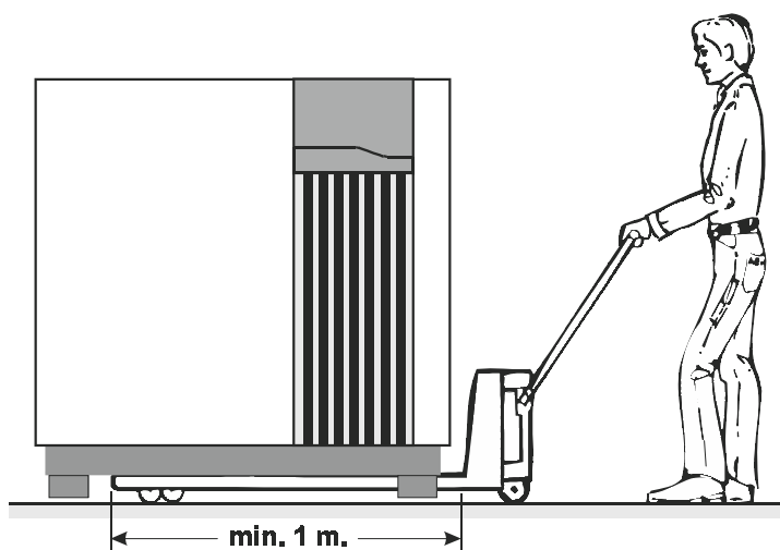
Рис. 6 Перемещение котла.
