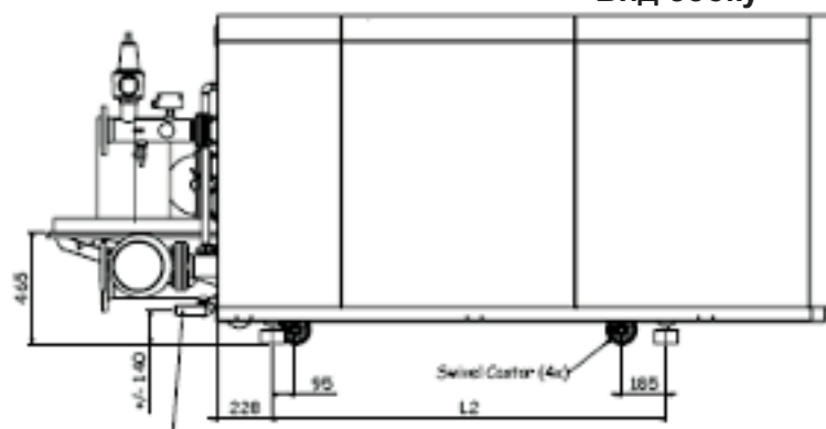
Вид сбоку
